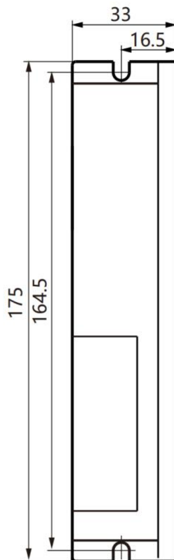
侧面安装
