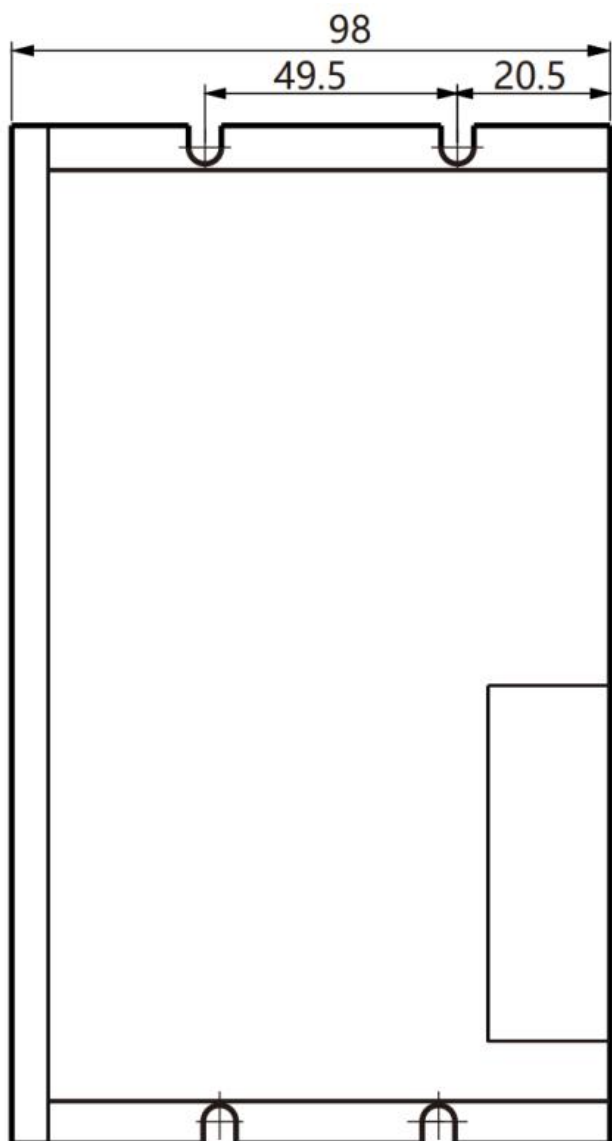
正面安装
