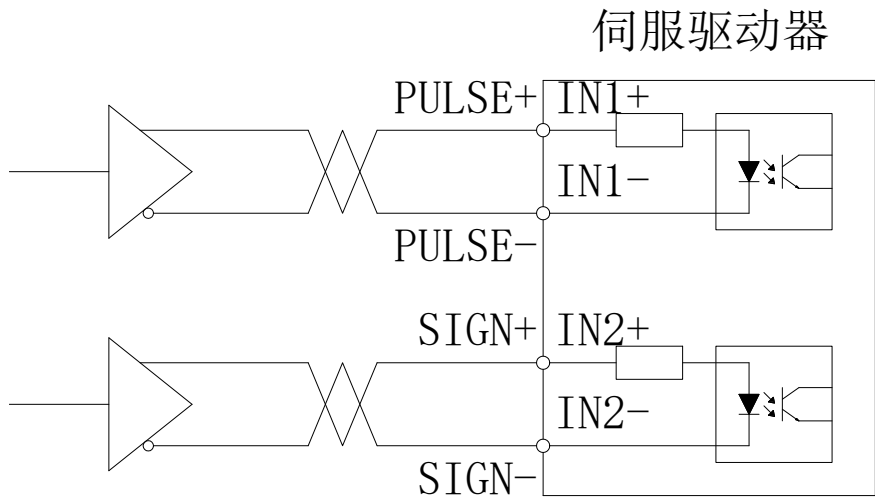
(b) 5V 单端输入
