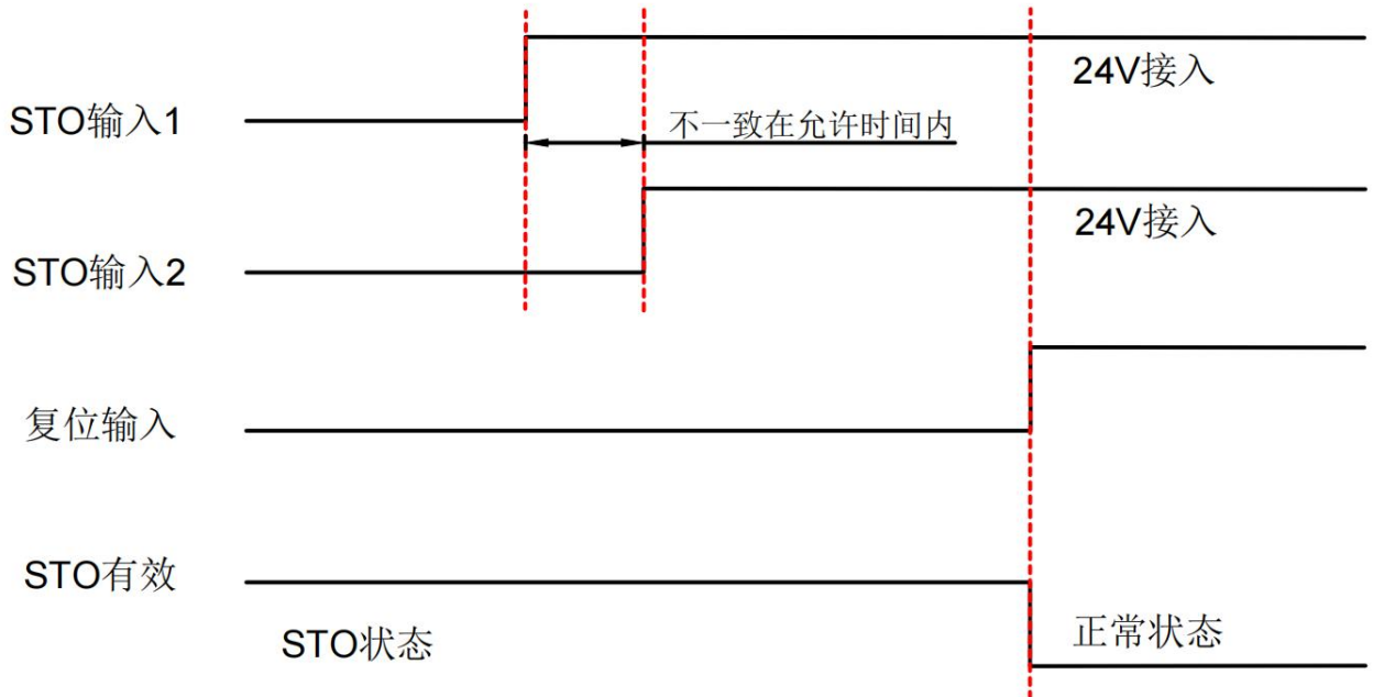
(2) 退出 ST0 安全状态的复位时序
